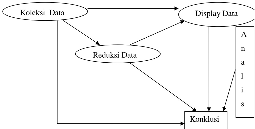
Gambar 1. Langkah-Langkah Penelitian
